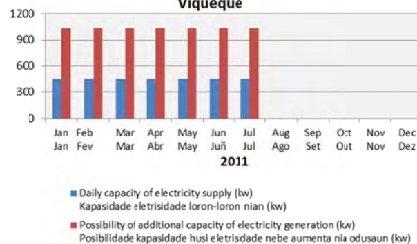
Electricity (kw) Supplied by EDTL Viqueque Fornesimentu (kw) Eletrisidade EDTL iha Viqueque
